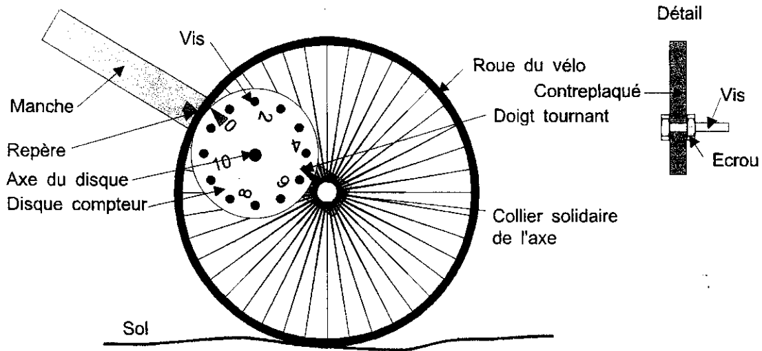
Schéma du "curvimètre"
