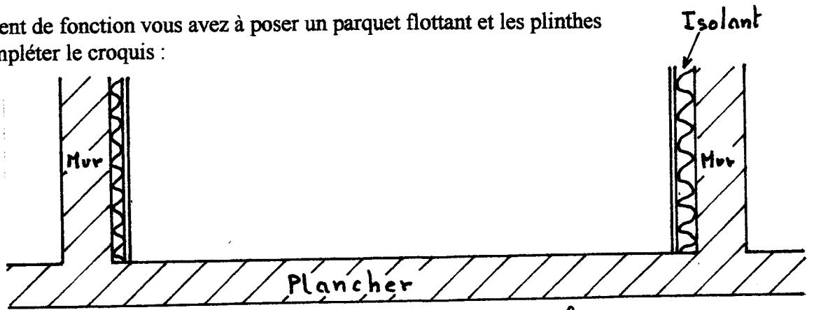
Coupe Verticale
